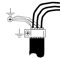
单屏蔽电缆
