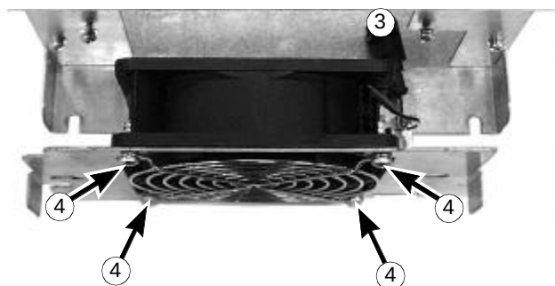
从上部看 风机安装板拉出
