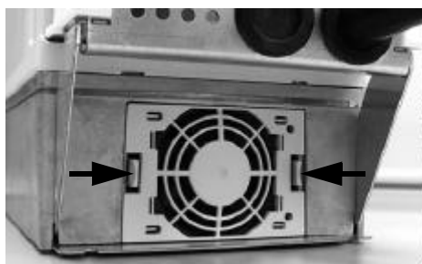
仰视图
