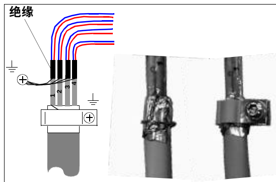
双屏蔽电缆
