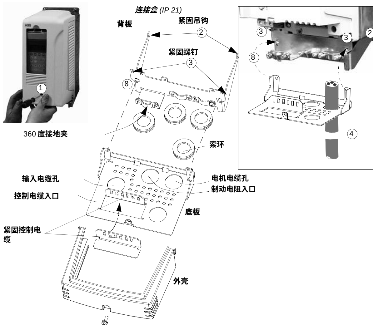
外形规格 R2 至 R4
