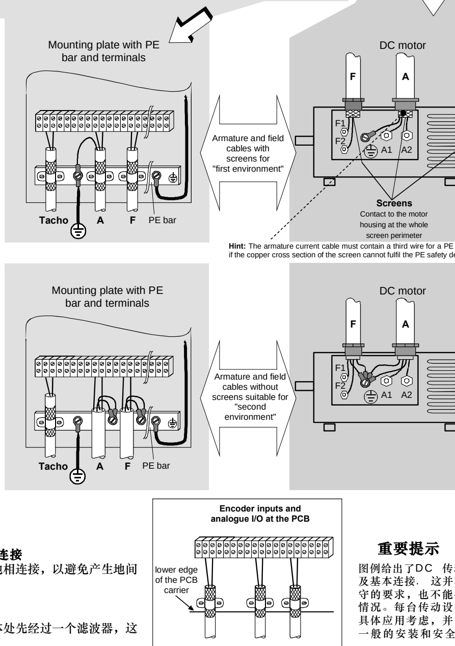
图 5.2.4 符合电磁兼容性要求的连接方式
