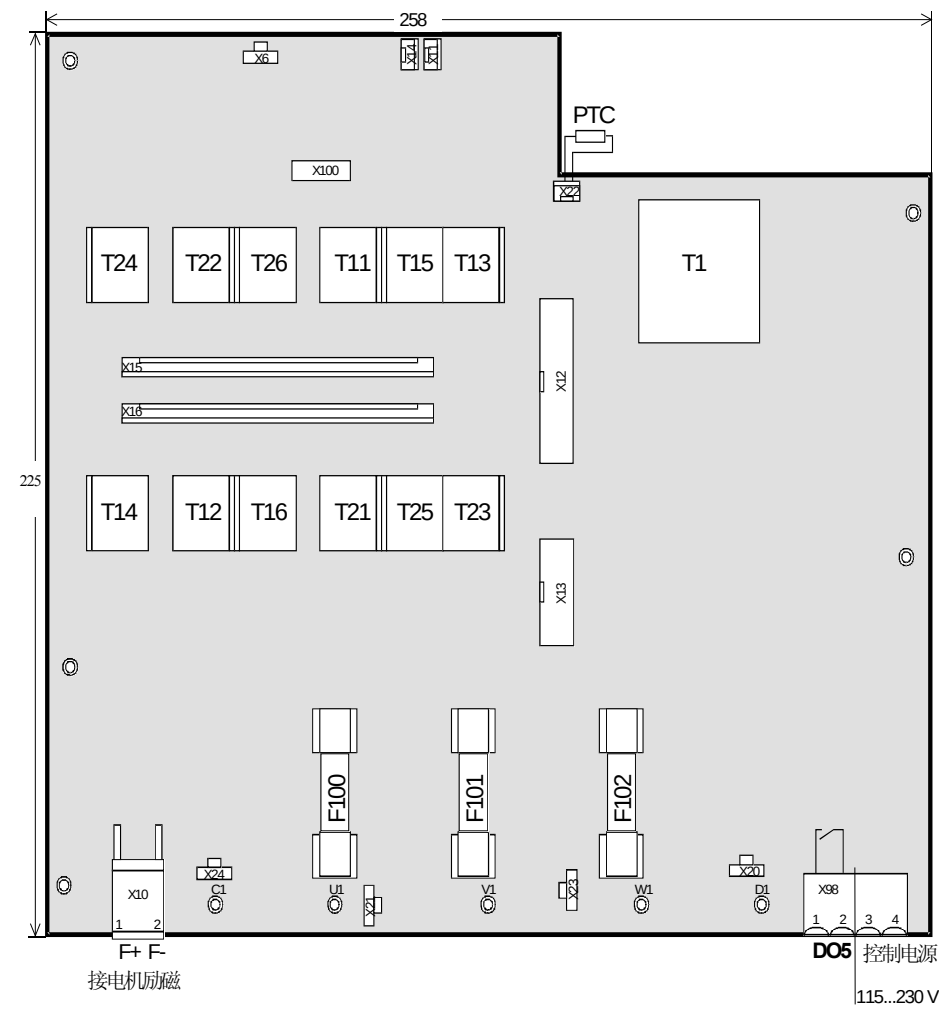
图 3.6.1 SDCS-PIN-3A 板布局图。
