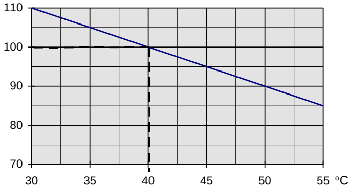
图 2.1.2: 环境温度对变流器负载能力的影响。
